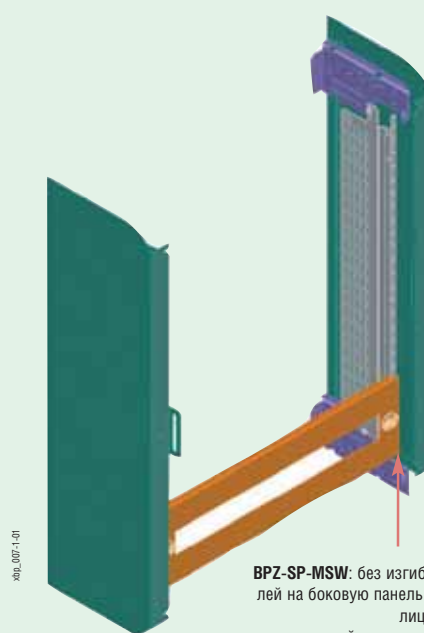
BP-SP: изгиб для монтажа лицевых панелей, нельзя комбинировать с боковой стенкой ВРZ-MSW
