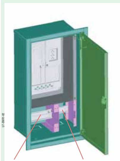
Приборная рейка для неизмеряемой части (8 модулей)
